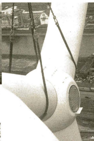
6) Die Montage des Rotors stellte eine besondere Herausforderung an Mensch und Maschine dar
