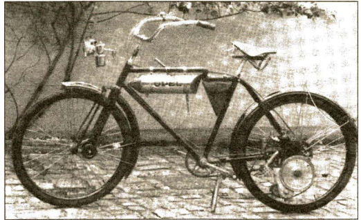
OPEL, Baujahr 1913, 140ccm, 1 PS Besitzer: Armin Weber
