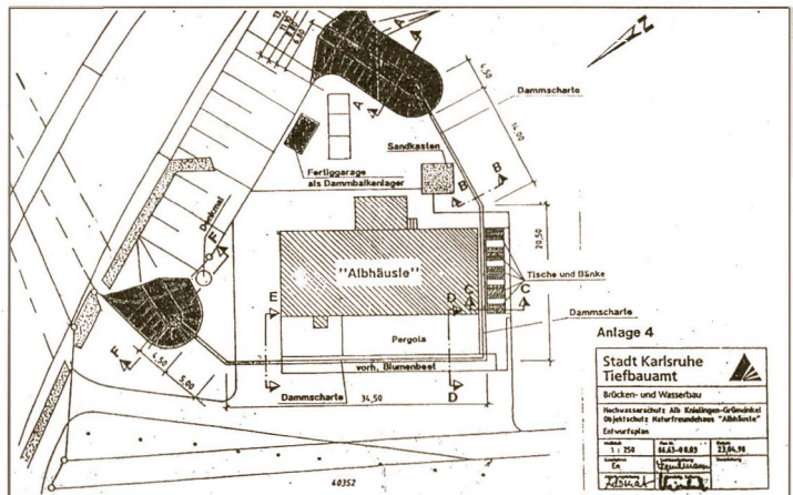
Planungsskizze: vorgesehener Hochwasserschutz am Naturfreundehaus „Albhäusle“
