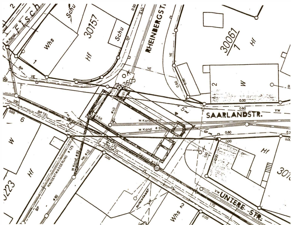
Neubau eines Regenüberlaufbeckens
