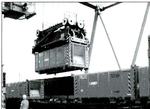
Bahnverladung der Müllsammelbehälter für den Transport zur Müllverbrennung nach Mannheim
